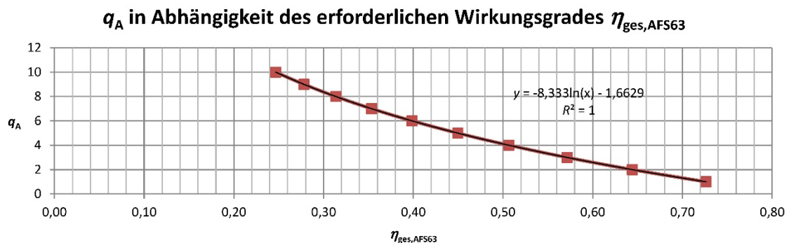
Bild 4: Abgeleitete Regressionsbeziehung zwischen Gesamtwirkungsgrad \eta_{ges,AFS63} und Bemessungswert der Oberflächenbeschickung q_{A,Bem}
