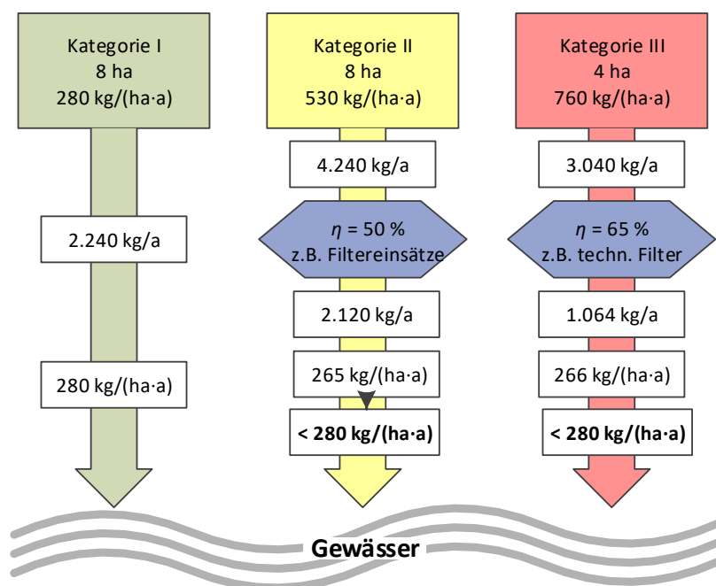
Bild 2: Schematische Darstellung der Entwässerungssituation bei getrennter dezentraler Behandlung der behandlungsbedürftigen Abflüsse der Belastungskategorien II und III mit jeweils eigener Einleitstelle
